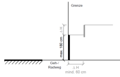
Strasse mit Geh- und / oder Radweg
