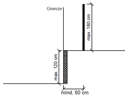
Stützmauern mit Einfriedungen
