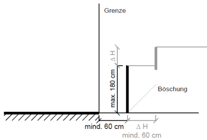
Strasse ohne Geh- und / oder Radweg
