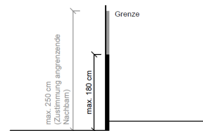
Einfriedungen
