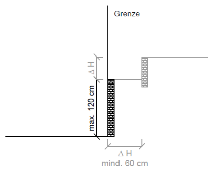
Stützmauern
