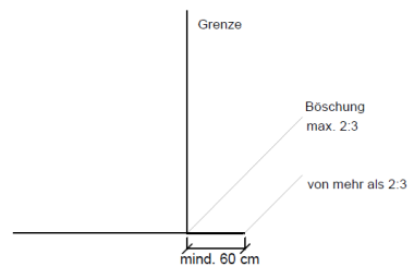
Böschungen (§ 28 BauV)
