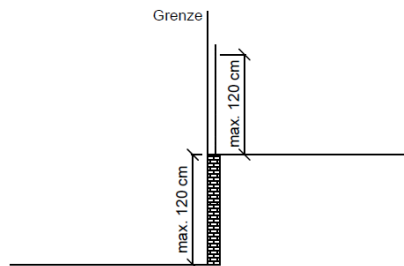
Stützmauern mit Schutzgeländer
