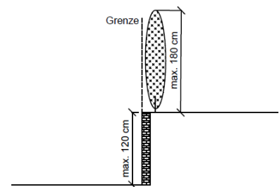
Stützmauern mit Bepflanzung
